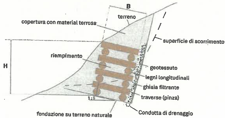
Schizzi sistema vista frontale (sopra) e sezione (sotto).
