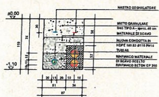
SEZIONE 2 - 2 SU STRADA STERRATA 1:20
