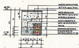
SEZIONE 3 - 3 SU STRADA ASFALTATA 1:20
