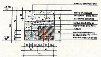
SEZIONE 2 - 2 SU STRADA STERRATA 1:20
